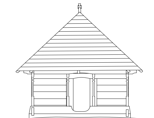
Fațadă vest sc. 1:100
