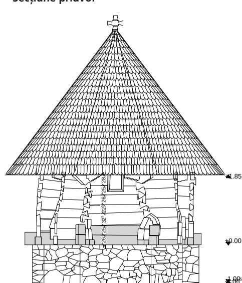
Fațadă vest
