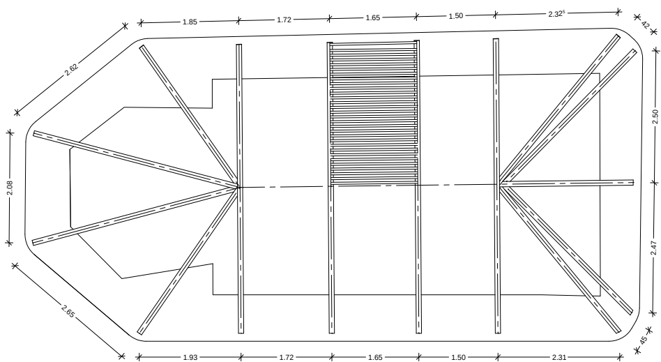
Plan căpriori
