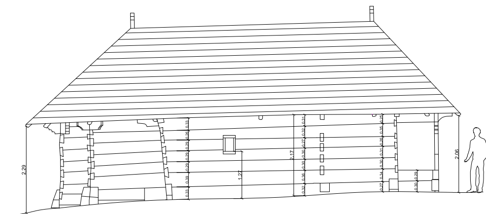
Fațadă nord sc. 1:100
