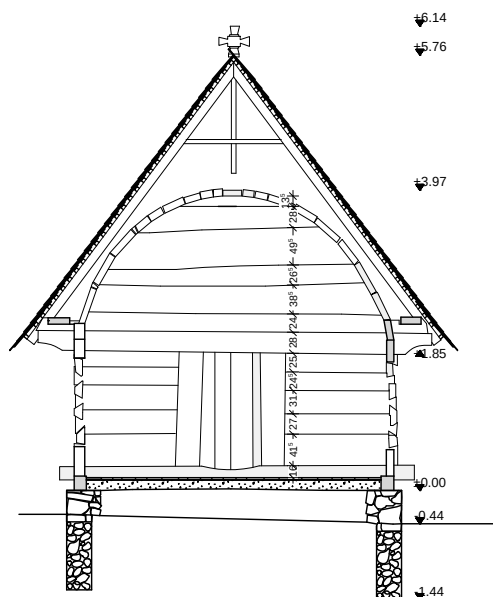
Secțiune pridvor
