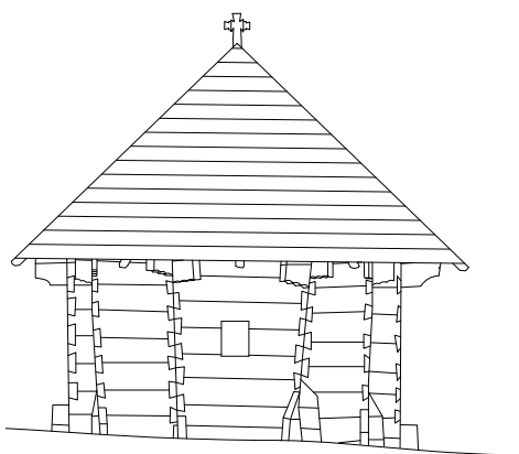
Fațadă est sc. 1:100
