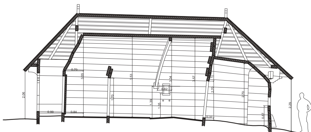
Secțiune sc. 1:100
