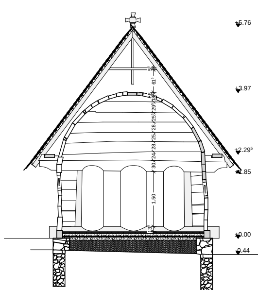
Secțiune naos
